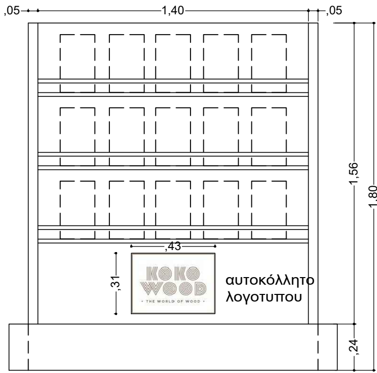
ΟΨΗ
