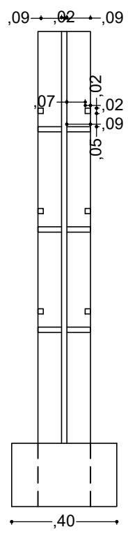
ΤΟΜΗ
